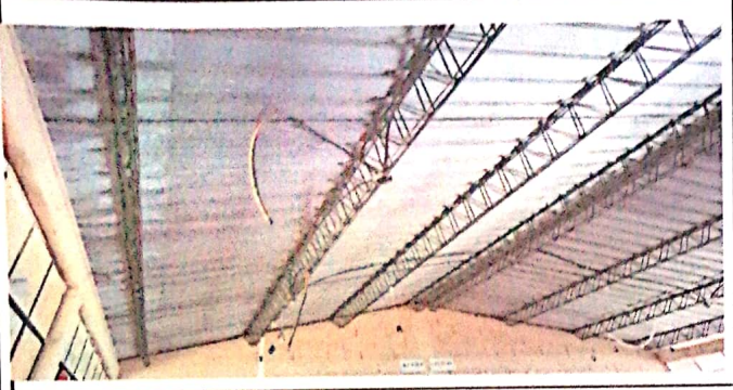
Foto1: Sustitucion de varillas de hierro por Costanera Galvanizadas.
